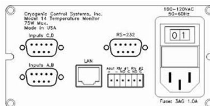
12 温度监视器后面板
